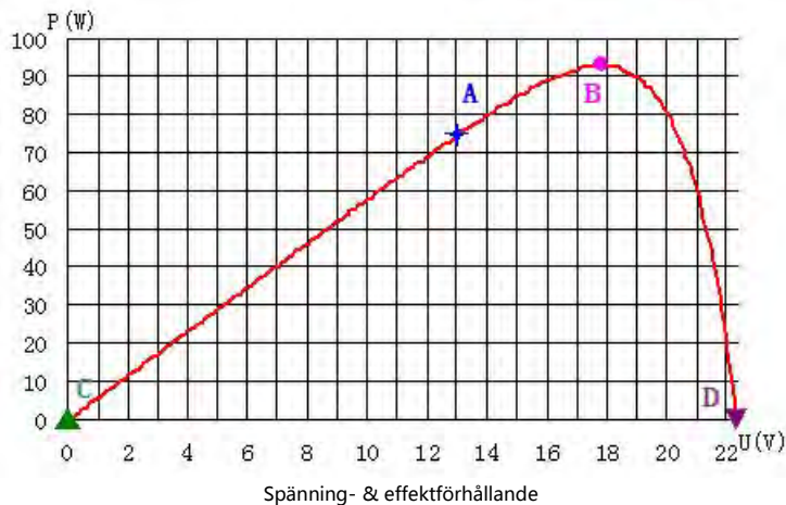
Spänning- & effektförhållande
